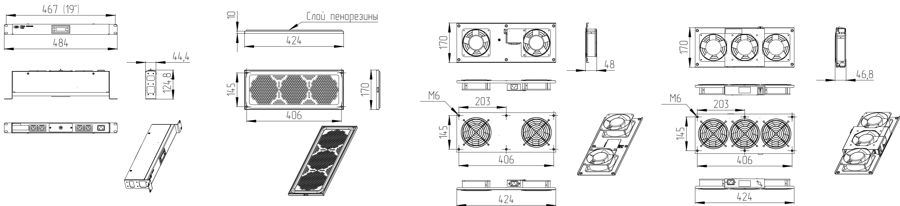
Фильтр MB-Ф
