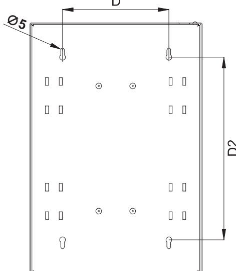
ВИД СЗАДИ
